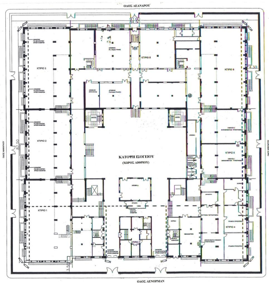
ΚΑΤΟΨΗ ΙΣΟΓΕΙΟΥ ΚΛΙΜΑΚΑ : 1: 500
