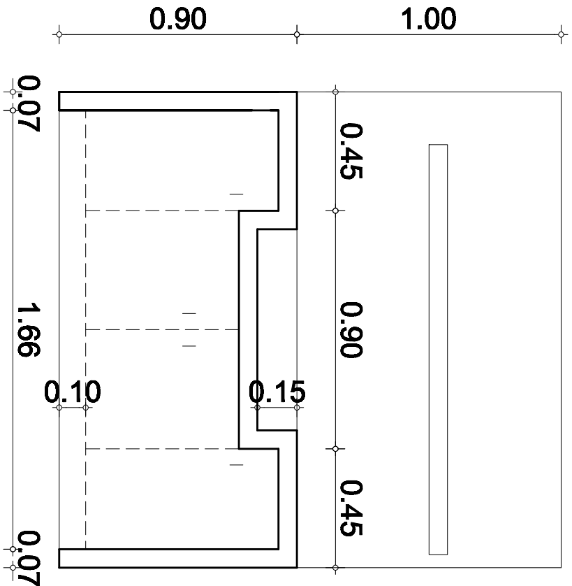
Τομή
