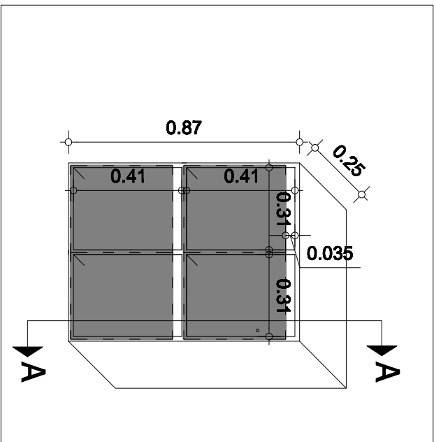
ΑΕΟΝΟΜΕΤΡΙΚΗ ΑΠΕΙΚΟΝΙΣΗ (4 ΘΥΡΙΔΕΣ) ΚΛΙΜΑΚΑ 1:20
