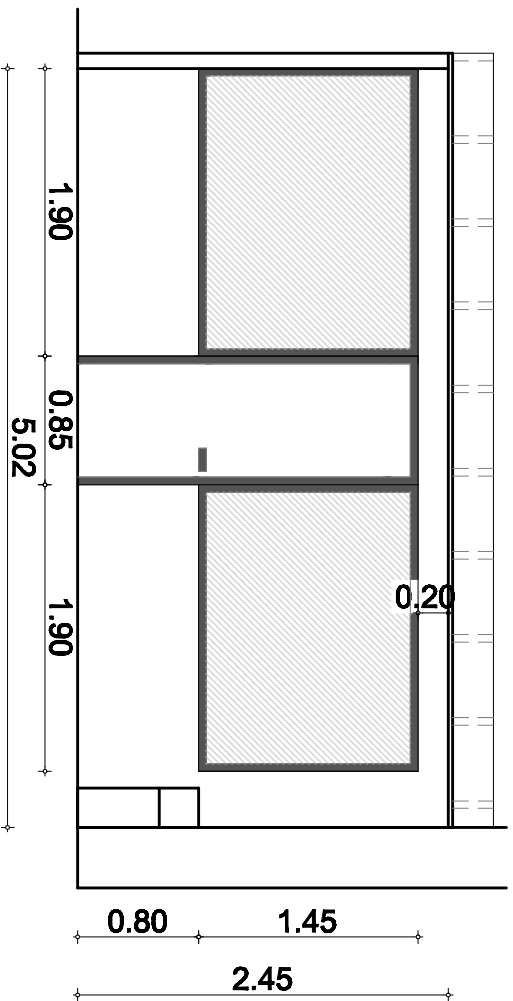
ΟΨΗ Β-Β
