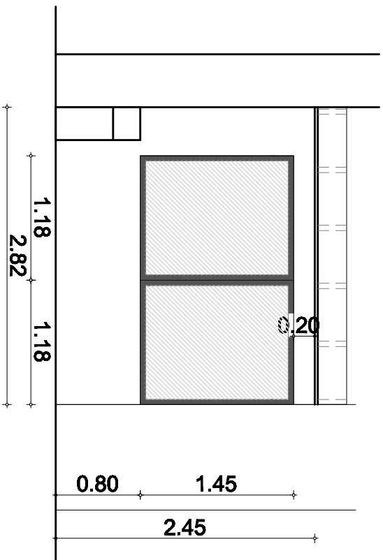
ΟΨΗ Δ-Δ
