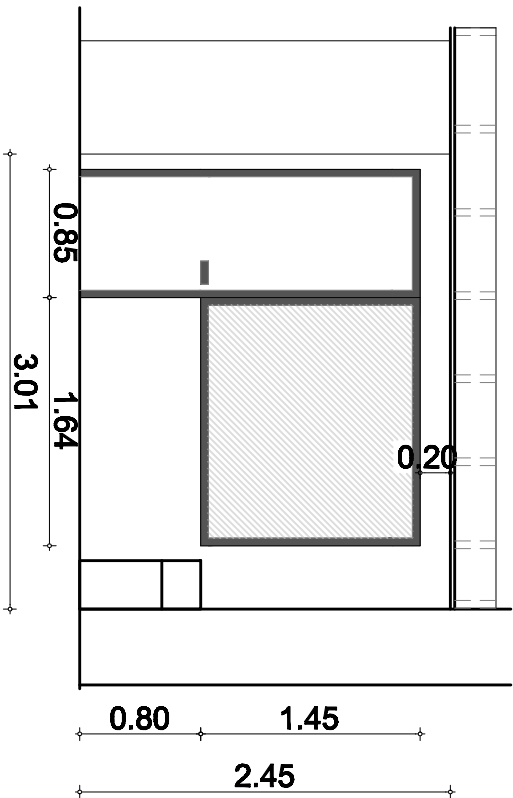
ΟΨΗ Γ-Γ
