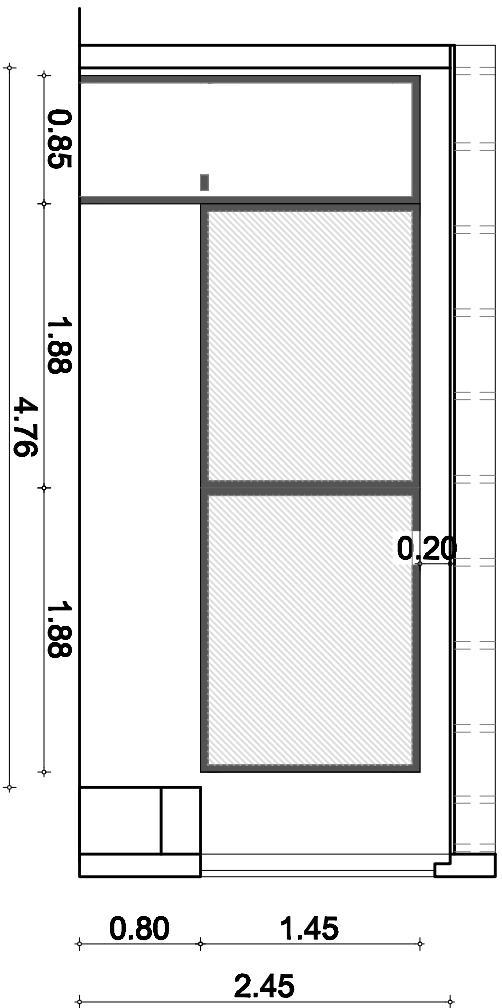
ΟΨΗ Α-Α
