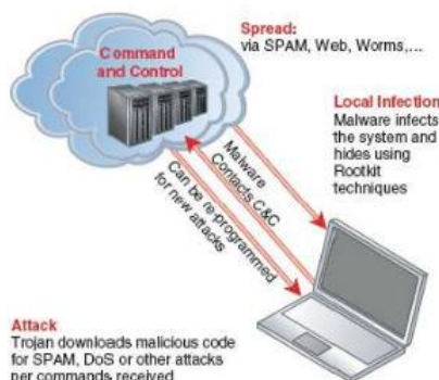
Σχήμα 1: Bot attack
