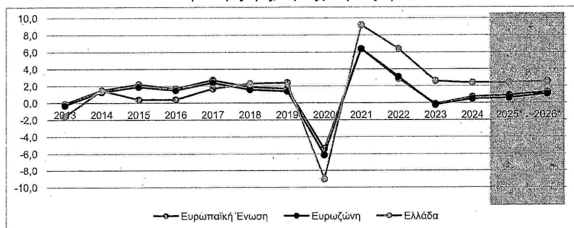
Διάγραμμα 1.9.: Ρυθμός μεταβολής κατά κεφαλήν ΑΕΠ (σταθερές τιμές, ετήσιες μεταβολές %)
