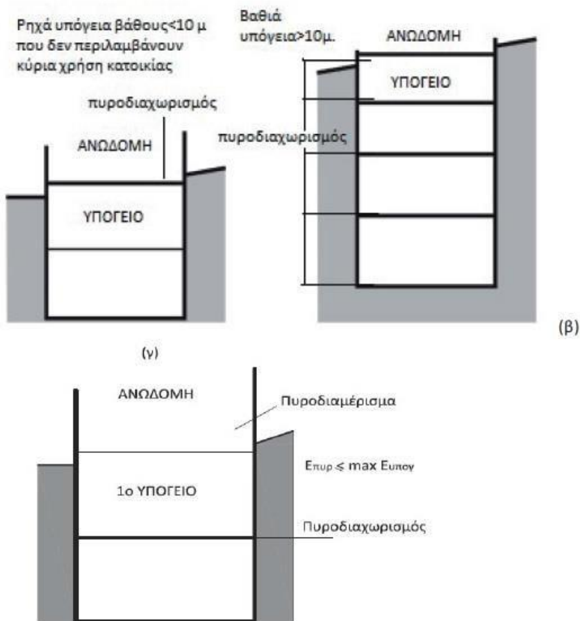
Σχήμα 16: Πυροδιαχωρισμός υπογείων
