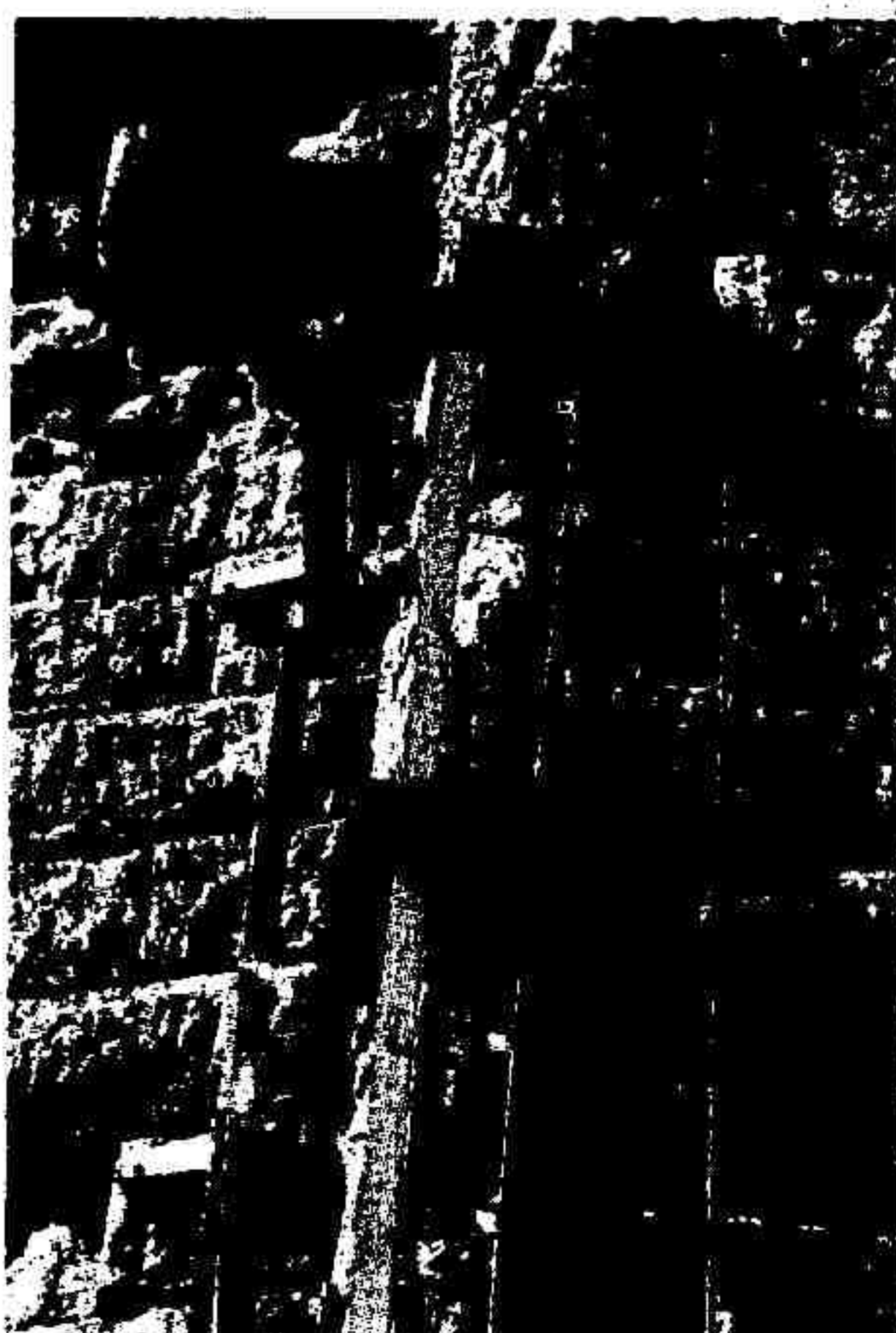
Εάν δεν τοποθετηθούν νέες ντιζες, το κομμάτι του τείχους είναι έτοιμο να καταρρεύσει βάζοντας σε κίνδυνο και τους αμέρηνους επισκέπτες
