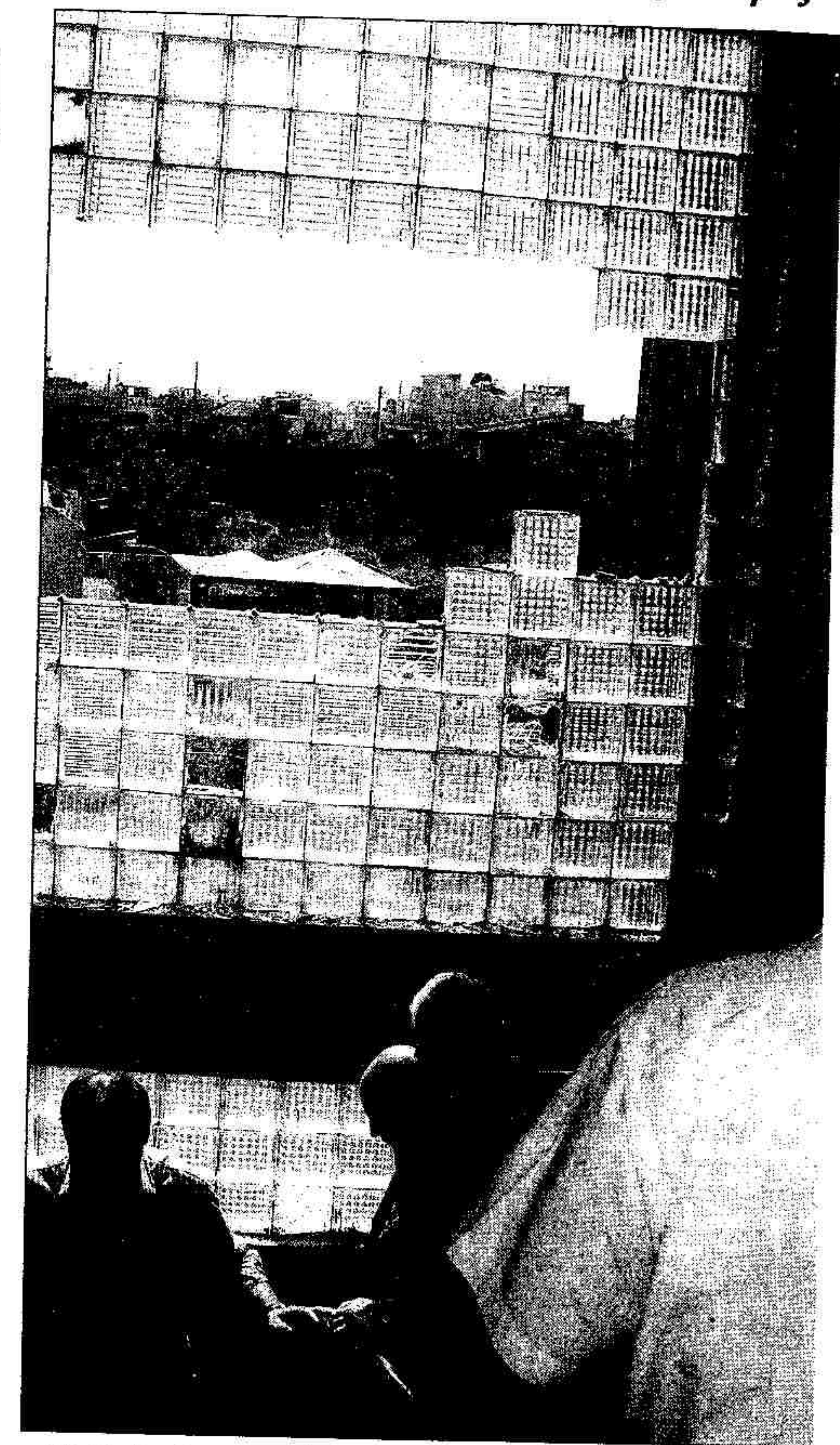
Τα σχολικά συγκροτήματα στην Κ. Αχαΐα, όπου εντοπίστηκε το επίκεντρο του ισχυρού σεισμού της 8ης Ιουνίου του 2008, είχαν υποστεί πολύ σοβαρές και εκτεταμένες ζημιές
