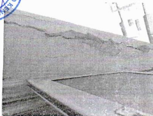
Φ.3 & Φ.4 Έντονη οξείδωση σιδηροπλισμού με φουσκώματα, ρηγματώσεις και χαλαρά τμήματα επικάλυψης σιδηροπλισμού επικινδύνου προς αποκόλληση κυρίως σε πρέκια παραθύρων επί της οδού Ψαρρού (στενός δρόμος).
