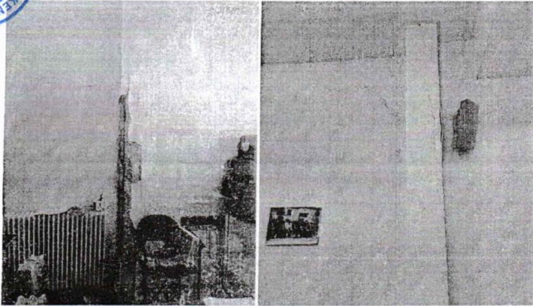
Φ.8 & Φ.9 Φουσκώματα, ρηγματώσεις και αποκόλληση επιχρισμάτων και επικάλυψης σιδηροπλισμού με έντονη οξείδωση σιδηροπλισμού στο εσωτερικό του ισόγειου του κτιρίου (χρησιμοποιείται από το Εργατικό Κέντρο Ρεθύμνου).
