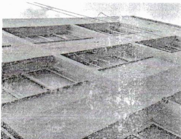
Φ.5 & Φ.6 Εκτεταμένα προβλήματα όπως Φ.3.&Φ.4 σε οριζόντια και κατακόρυφα στοιχεία οπλισμένου σκυροδέματος επί της οδού Ψαρρού
