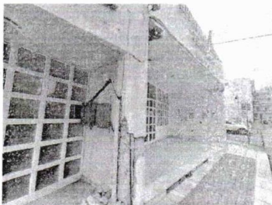
Φ.7 & Φ.8 Ρηγματώσεις και αποκόλληση επιχρισμάτων και επικάλυψης σιδηροπλισμού με έντονη οξείδωση σιδηροπλισμού σε κατακόρυφο στοιχείο και στην πρόσοψη της εισόδου του Εργατικού Κέντρου Ρεθύμνου επί της Πλατείας Προτομαγιάς
