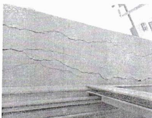
Φ.3 & Φ.4 Έντονη οξείδωση σιδηροπλισμού με φουσκώματα, ρηγματώσεις και χαλαρά τμήματα επικάλυψης σιδηροπλισμού επικινδύνου προς αποκόλληση κυρίως σε πρέκια παραθύρων επί της οδού Ψαρρού (στενός δρόμος).
