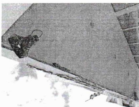
Φ.7 & Φ.8 Ρηγματώσεις και αποκόλληση επιχρισμάτων και επικάλυψης σιδηροπλισμού με έντονη οξείδωση σιδηροπλισμού σε κατακόρυφο στοιχείο και στην πρόσοψη της εισόδου του Εργατικού Κέντρου Ρεθύμνου επί της Πλατείας Προτομαγιάς
