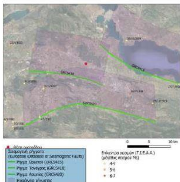
Σχήμα 8-12 Ευρώτερη περιοχή λόγω σε σχέση με τα ενεργά ρήματα της περιοχής (από ΕΔΣΕ, Ευρωπαϊκή Πύλη Δεδομένων Σεισμολογικών Πληροφοριών επί επίκεντρα σεισμών (από Γεωλογικό Ινστιτούτο Εθνικού Αστεροσκοπείου Αθηνών)
