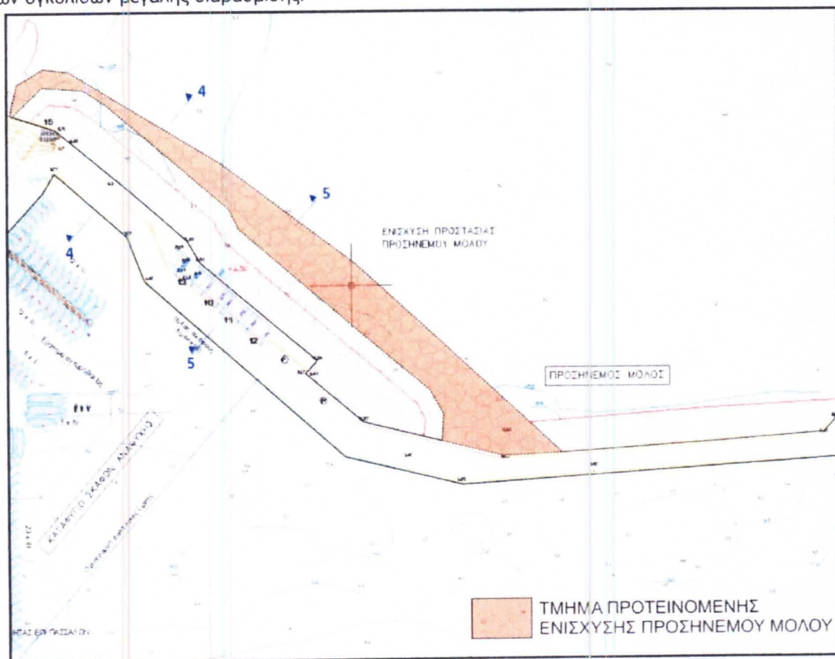
Σχέδιο 1. Το τμήμα του προσήνεμου μόλου όπως προτείνεται η ενίσχυσή του, στην μελέτη “Πλαίσιο έργων ανάπτυξης λιμένα Σκοπέλου”.
