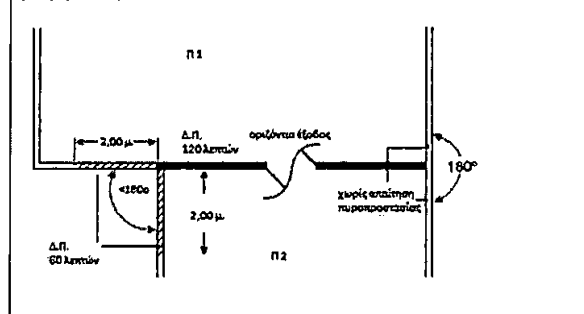
Σχήμα 24: Επέκταση πυραντίστασης τοίχων πυροδιαμερισμάτων που επικοινωνούν με οριζόντια έξοδο
