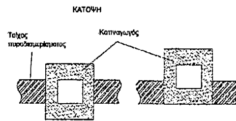
Σχήμα 21: Τυπική διάταξη πυράντοχων διαφραγμάτων (damper)
