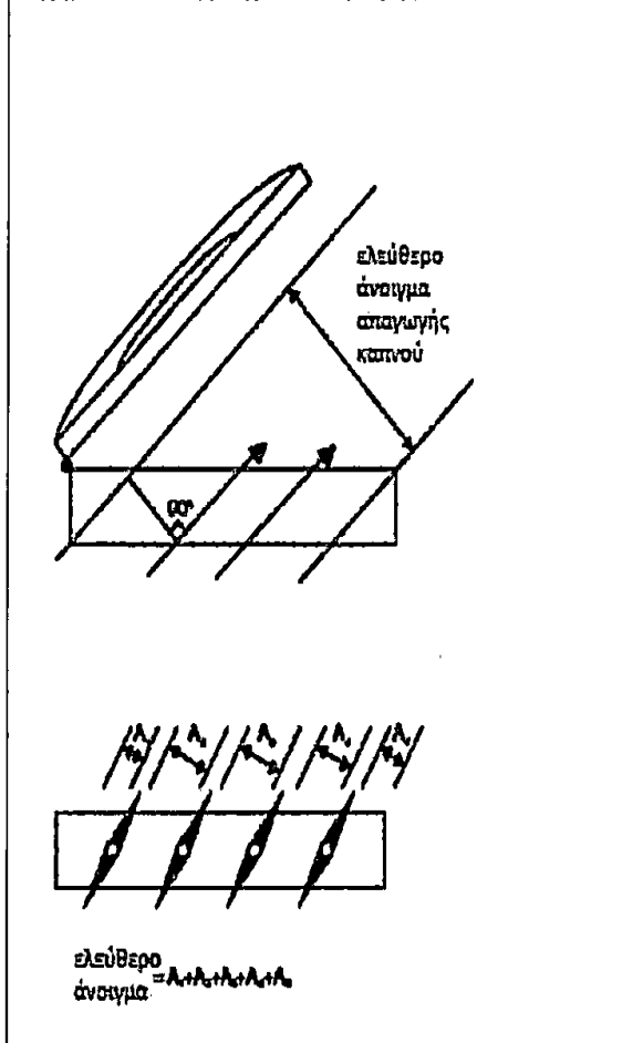
Σχήμα 22: Διάφραγμα απαγωγής καπνού
