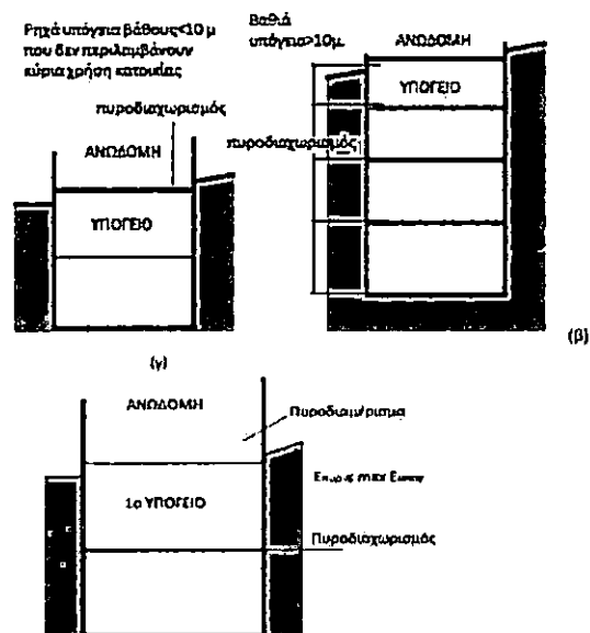
Σχήμα 16: Πυροδιαχωρισμός υπογείων
