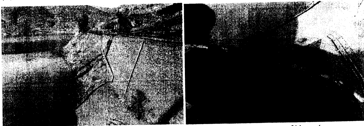
Φωτ. Ε.3.1, Ε.3.2: Μερικό σύστημα συλλογής ομβρίων σε τσιμεντένιες πλατφόρμες στις προβλήτες φόρτωσης.
