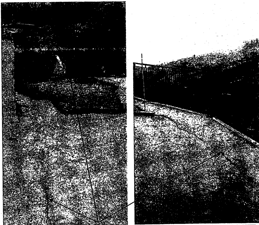
Φωτογραφίες 4 και 5 ρηγμάτωση του σκυροδέματος διάστρωσης και της περίφραξης
