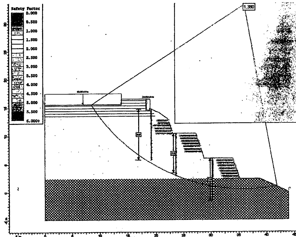
Σχήμα 6.4: Κύκλος ολίσθησης στην Τομή B-B
