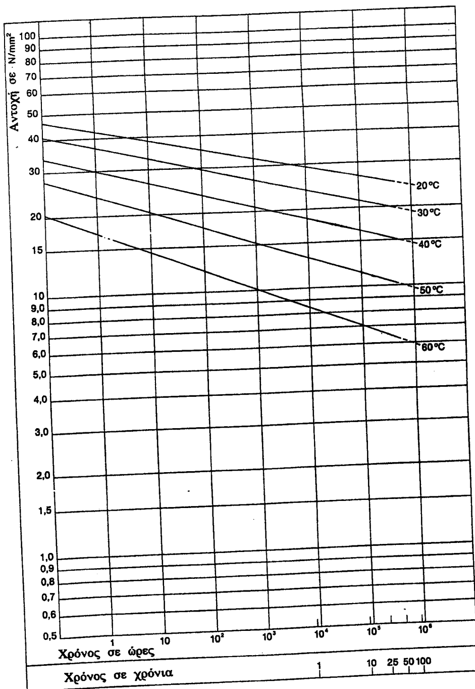
Σχήμα 7.9. Μεταβολή της αντοχής των σωλήνων από μη πλαστικοποιημένο χλωριούχο πολυβινύλιο συναρτήσει του χρόνου και της θερμοκρασίας.
