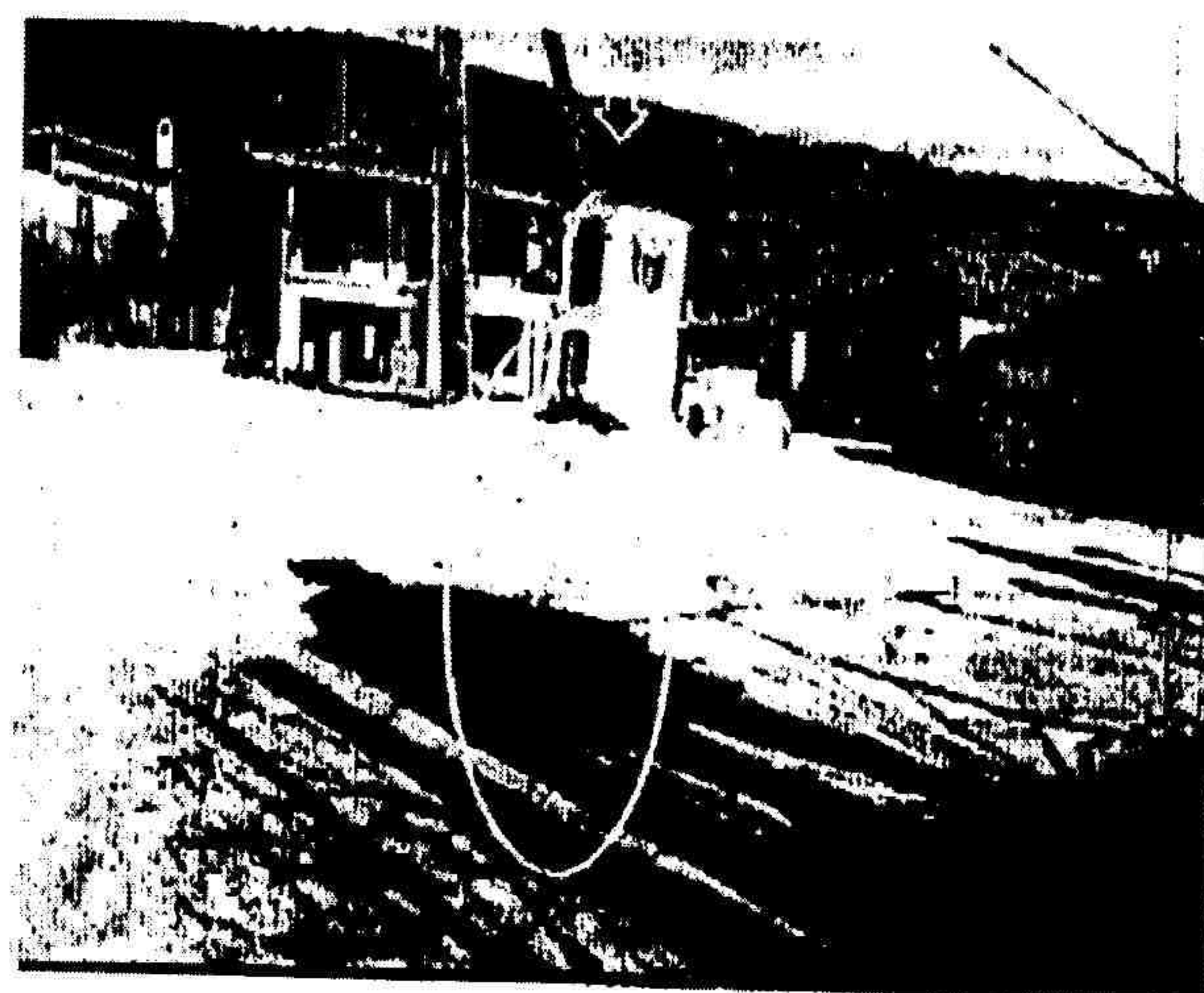
Φωτο. 1&2: Ρηγμάτωση - ανύψωση - αποδιοργάνωση πλακόστρωτου και απόκλιση από το κατακόρυφο της κολώνας και του παρεκκλησίου αντίστοιχα (θέση 1)
