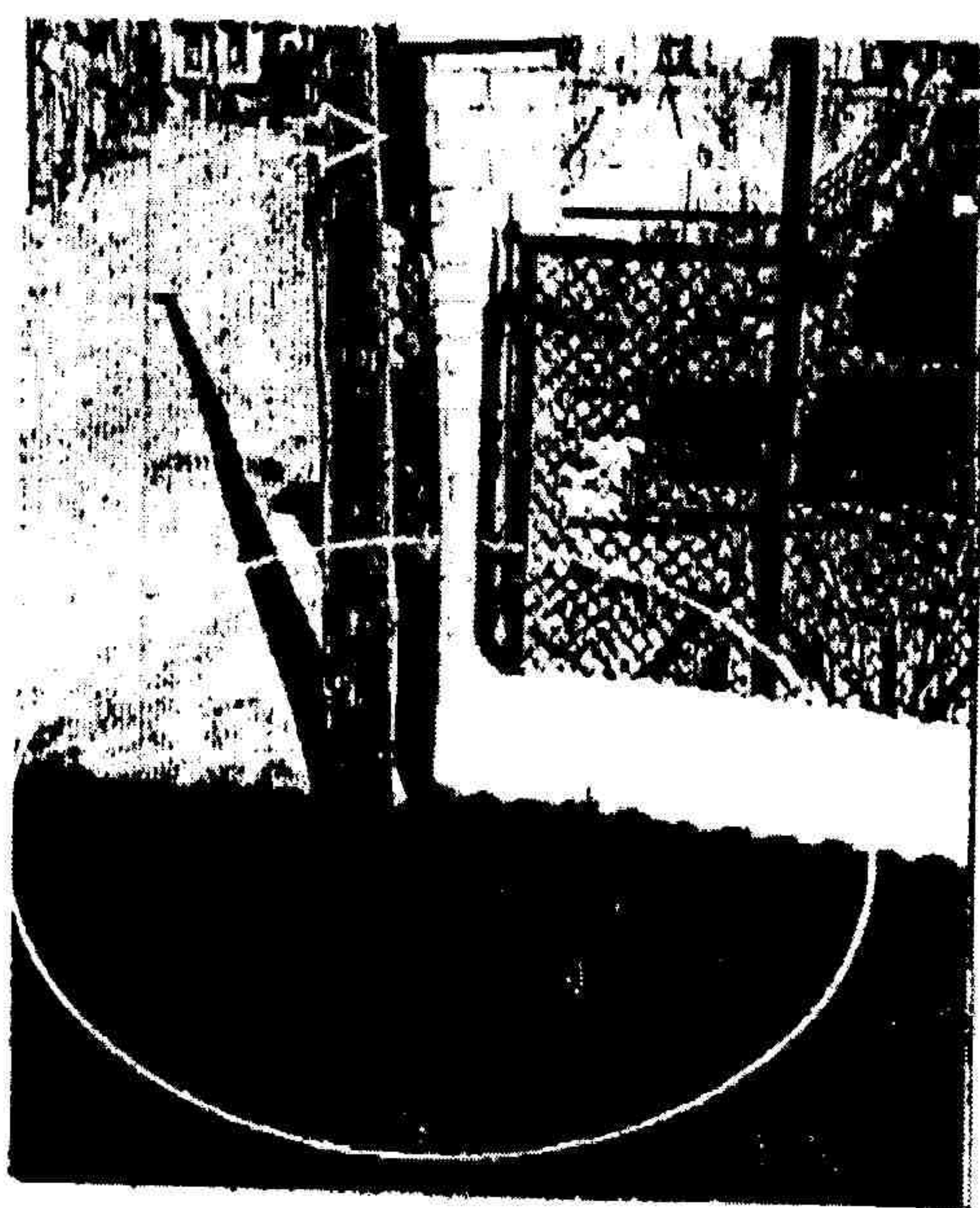
Φωτο. 1&2: Ρηγμάτωση - ανύψωση - αποδιοργάνωση πλακόστρωτου και απόκλιση από το κατακόρυφο της κολώνας και του παρεκκλησίου αντίστοιχα (θέση 1)
