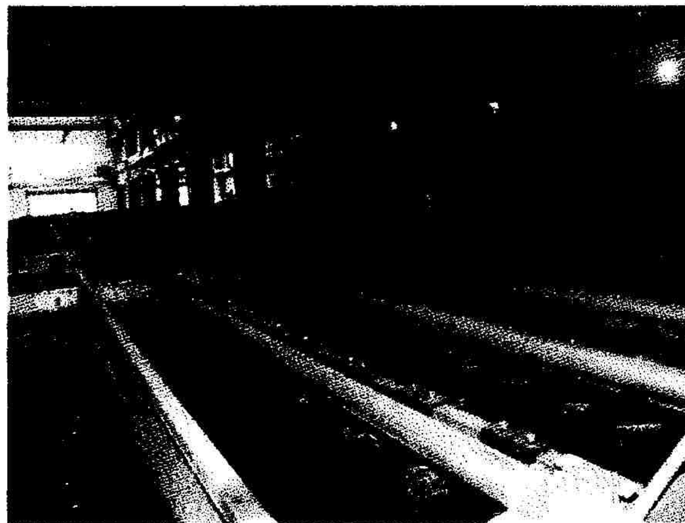
Φ.24 μηχανική πάχυνση βιολογικής λάσπης
