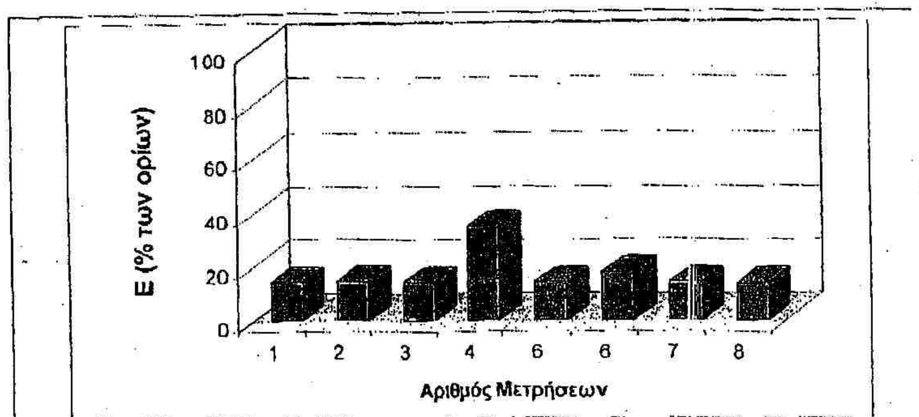
Σχήμα 4. Τιμές της έντασης του ηλεκτρικού πεδίου E, ως ποσοστό των ορίων έκθεσης του κοινού, όπως καταγράφηκαν σε όλες τις θέσεις μέτρησης.
