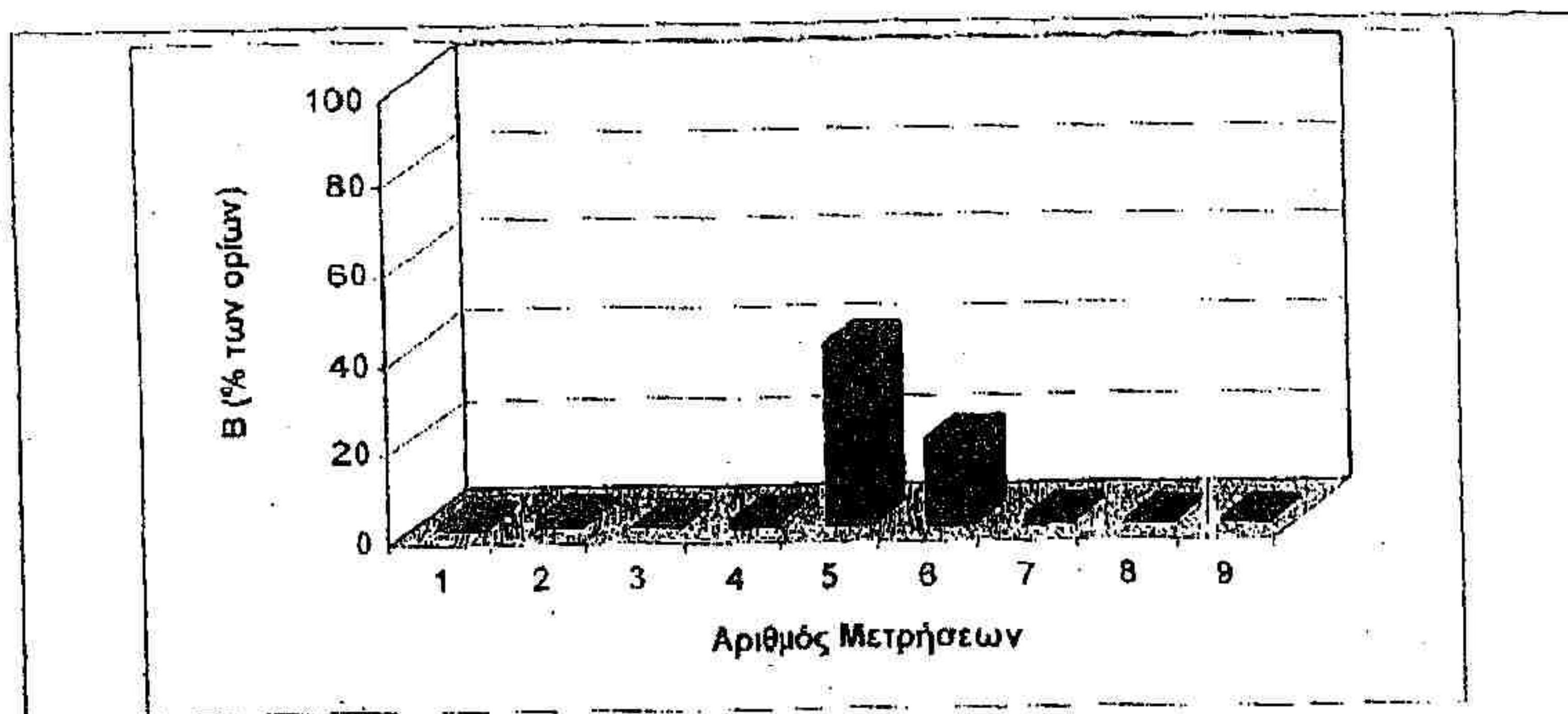
Σχήμα 3. Τιμές της μαγνητικής επαγωγής B, ως ποσοστό των ορίων έκθεσης του κοινού, όπως καταγράφηκαν σε όλες τις θέσεις μέτρησης.
