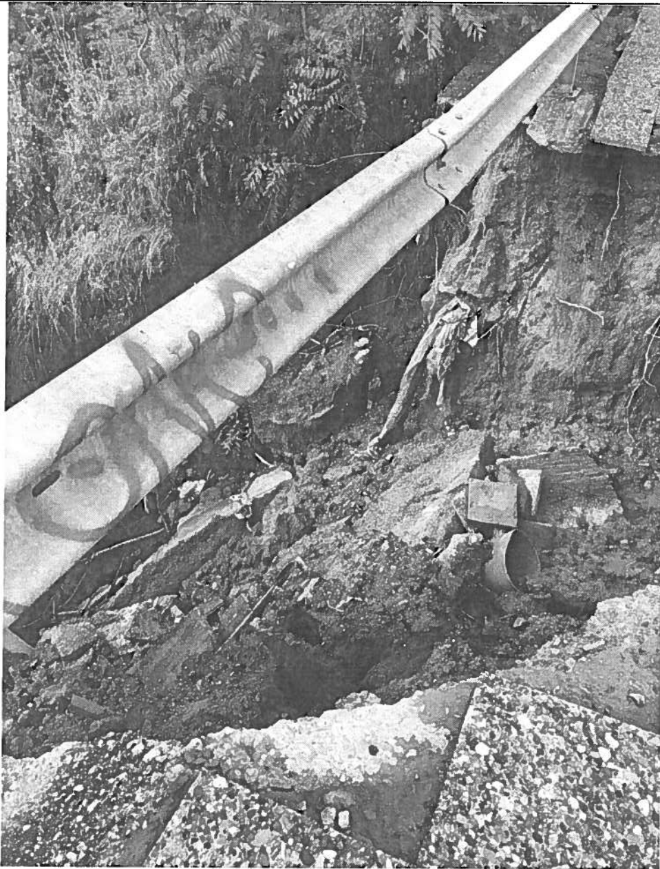
Εικόνα 2.1.6. Αποτυπώνεται η αστοχία επί του καταστρώματος της οδού Περικλέους, όπου έχει καταστραφεί το πεζοδρόμιο σε όλο το πλάτος του για μήκος περί τα 6,0-7,0μ., ο εγκιβωτισμένος αγωγός απορροής των ομβρίων και τοπικά το ανάντη τμήμα του επιχώματος έδρασης.
