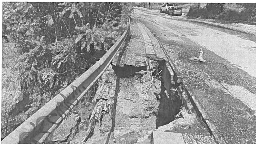
Εικόνα 2.1.4. Αποτυπώνεται η αστοχία επί του καταστρώματος της οδού Περικλέους, όπου έχει καταστραφεί το πεζοδρόμιο σε όλο το πλάτος του για μήκος περί τα 6,0-7,0μ., ο εγκιβωτισμένος αγωγός απορροής των ομβρίων και τοπικά το ανάντη τμήμα του επιχώματος έδρασης.
