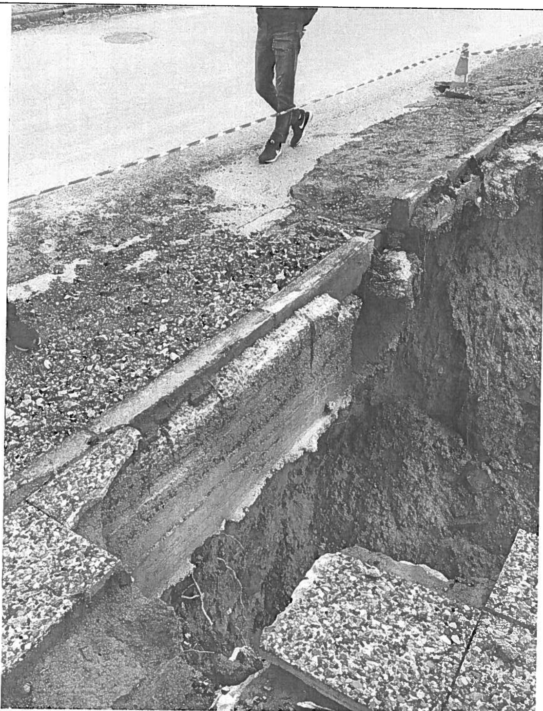
Εικόνα 2.1.5. Αποτυπώνεται η αστοχία επί του καταστρώματος της οδού Περικλέους, όπου έχει καταστραφεί το πεζοδρόμιο σε όλο το πλάτος του για μήκος περί τα 6,0-7,0μ., ο εγκιβωτισμένος αγωγός απορροής των ομβρίων και τοπικά το ανάντη τμήμα του επιχώματος έδρασης.
