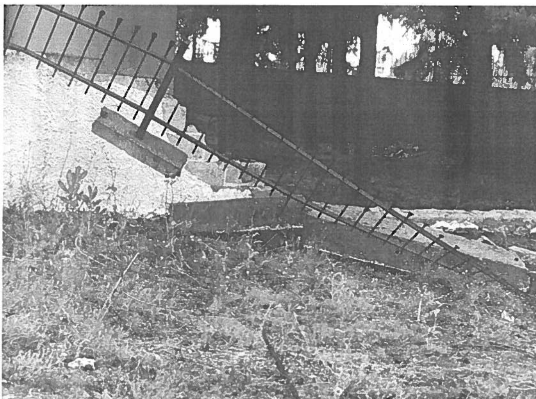
Εικόνα 19: Κατάρρευση περίφραξης Κοιμητηρίων Ταγαράδων
