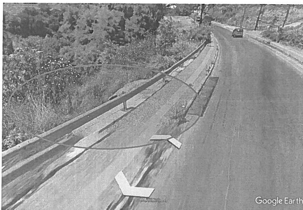
Εικόνα 2.1.3. Αποτύπωση θέσης αστοχίας με χρήση Google Earth (ημερομηνία εικόνας 7/2011). Παρουσιάζεται το υφιστάμενο τεχνικό έργο συλλογής και απορροής των ομβρίων στο χαμηλότερο μηκοτομικά σημείο της οδού και προς το ανάντη (σε σχέση με την ροή του ρέματος) πρανές του επιχώματος.
