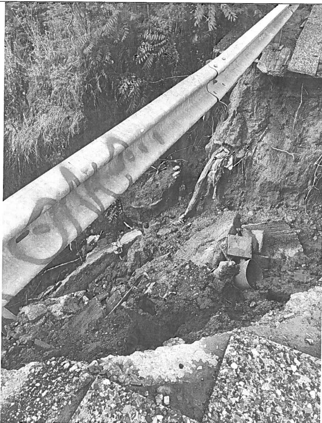
Εικόνα 2.1.7. Αποτυπώνονται κυρίως υλικά του αγωγού απορροής, τμήματος του καταστρώματος και πεζοδρομίου καθώς και του επιχώματος έδρασης, που έχουν αστοχήσει και κατολισθήσει σε τμήμα του ανάντη πρανούς.
