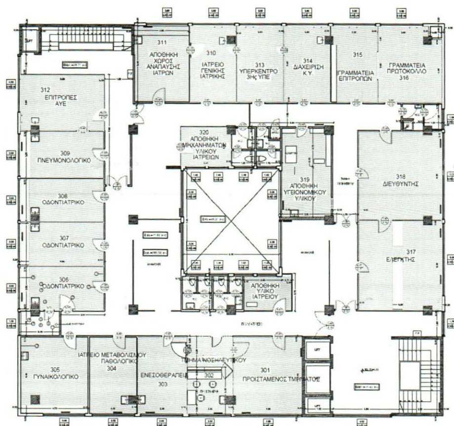
Κέντρο υγείας Πύλης Αξιού Κάτοψη 3ου ορόφου
