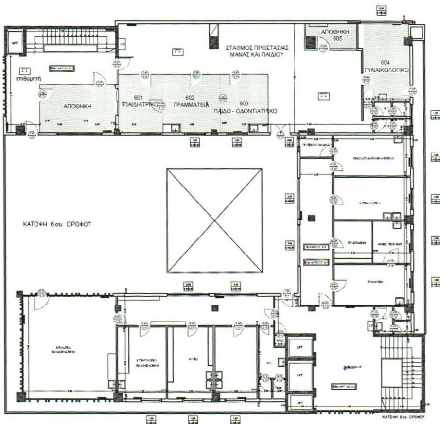
Κέντρο υγείας Πύλης Αξιού Κάτοψη 6ου ορόφου
