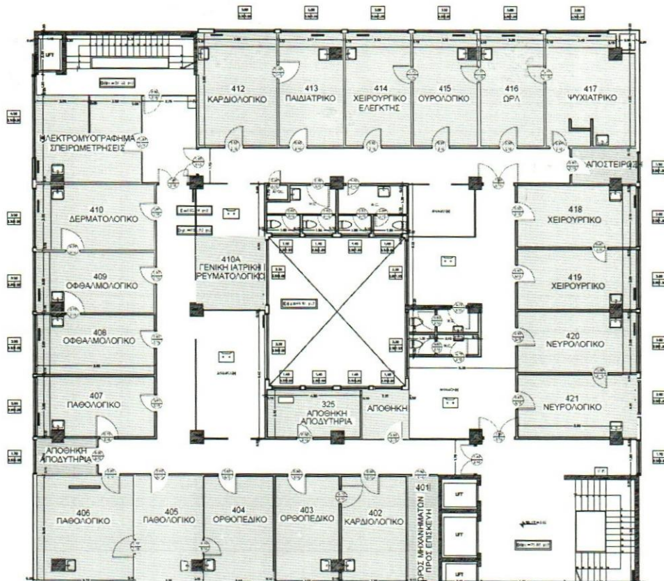
Κέντρο υγείας Πύλης Αξίου Κάτοψη 4ου ορόφου
