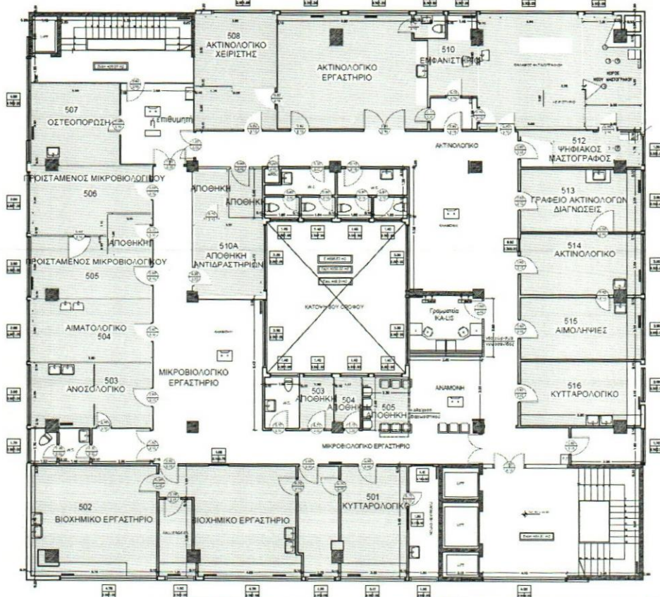
Κέντρο υγείας Πύλης Αξίου Κάτοψη 5ου ορόφου
