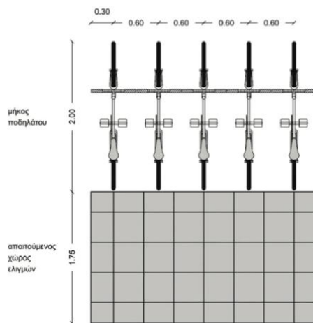
Σχήμα 1: διάταξη θέσεων σε σειρά
