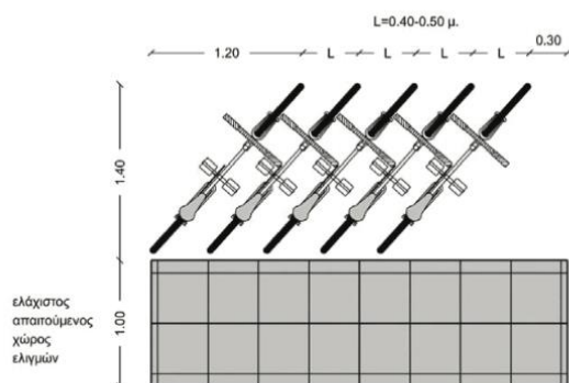
Σχήμα 2: διάταξη θέσεων υπό γωνία σε σειρά
