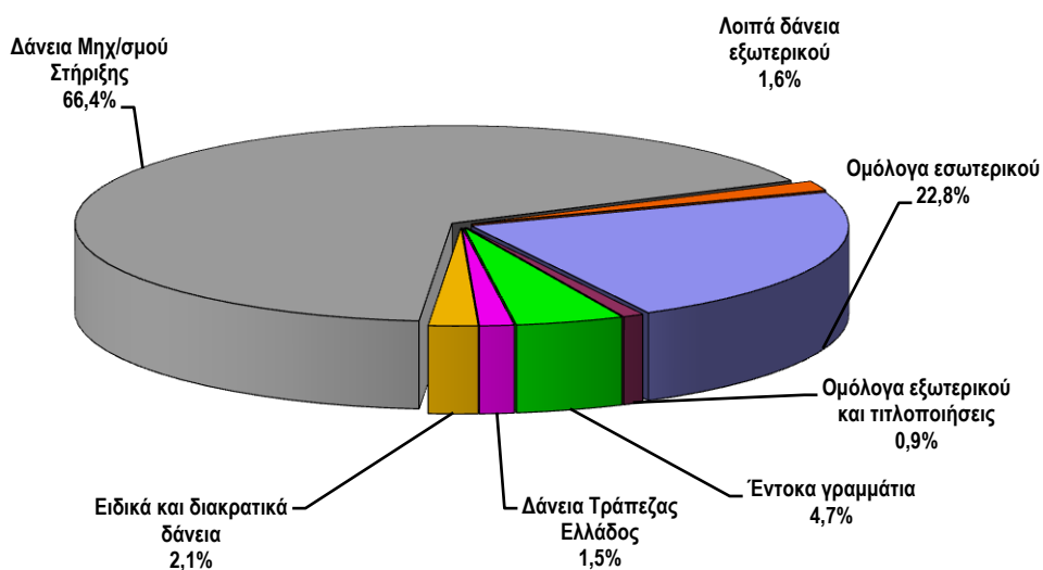
Διάγραμμα 4.2 Σύνθεση χρέους Κεντρικής Διοίκησης την 30/9/2013
